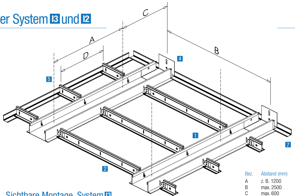
Sichtbare Montage, System 13
