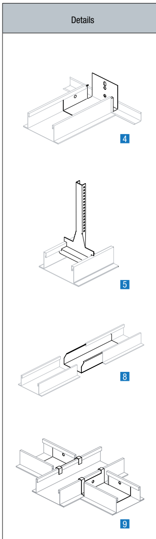
Halbverdeckte Montage, System 12
