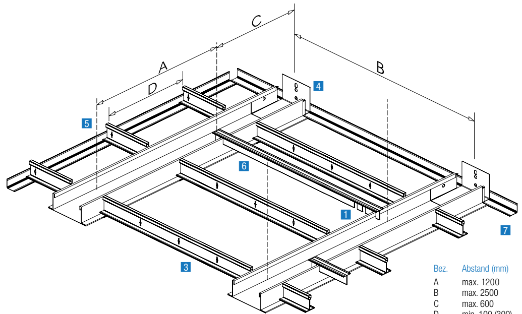
Halbverdeckte Montage, System 12
