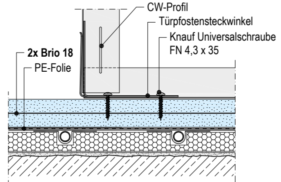
F128B.de-V28 Türpfostensteckwinkel
