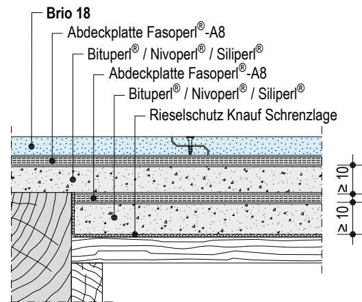
F126.de-V34 Höhenausgleich auf tragfähigem Fehlboden
