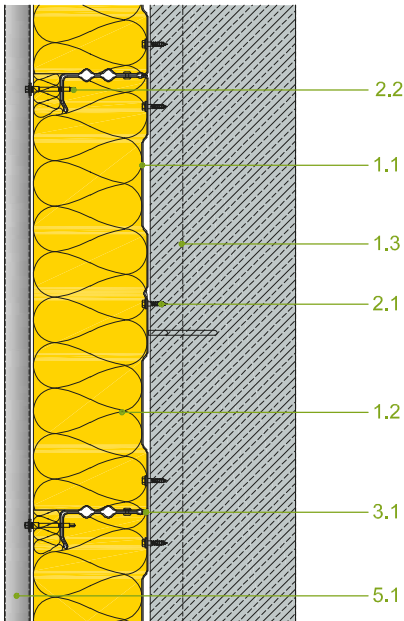
Kassettenwand mit nach unten gerichteten Kassettenobergurten
