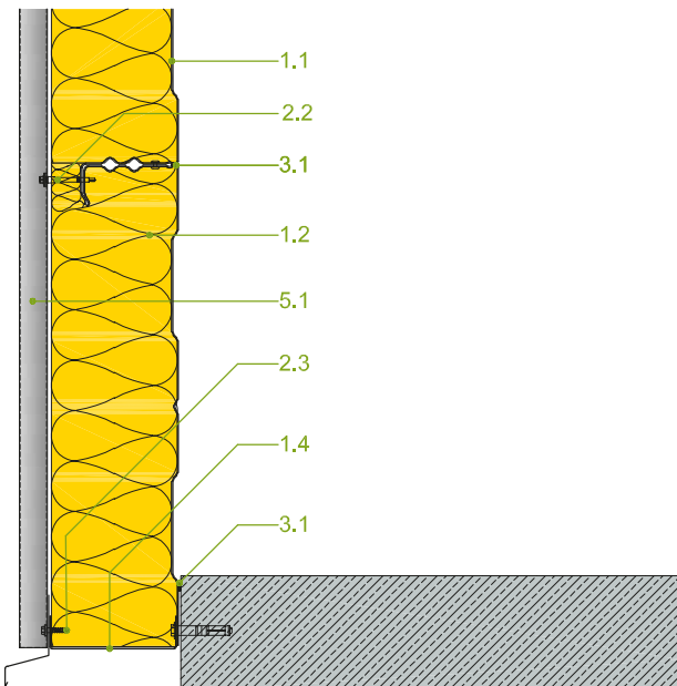
Sockelausbildung mit vorstehender Stahlkassette
