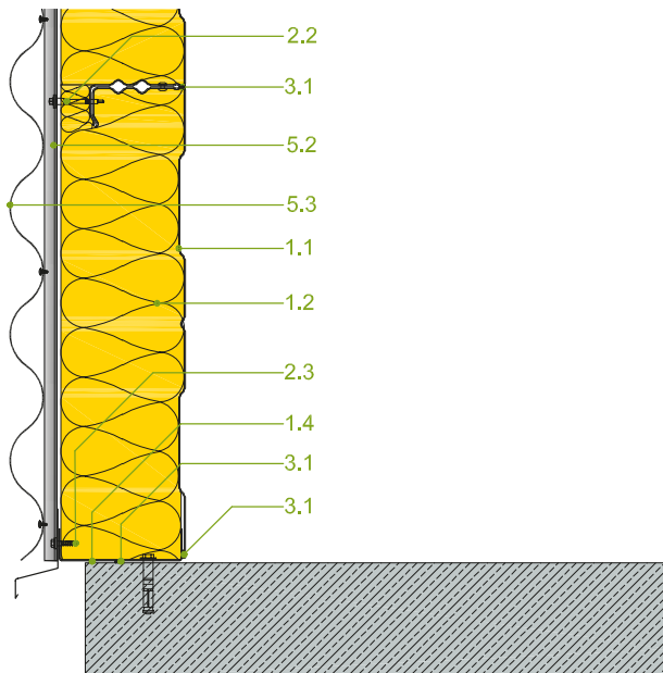
Sockelausbildung mit aufliegender Stahlkassette
