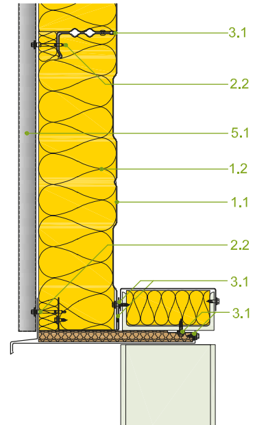
Oberer Toranschluss
