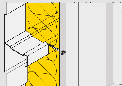
Möglich sind Schalldämmmaße von bis zu 51 dB
