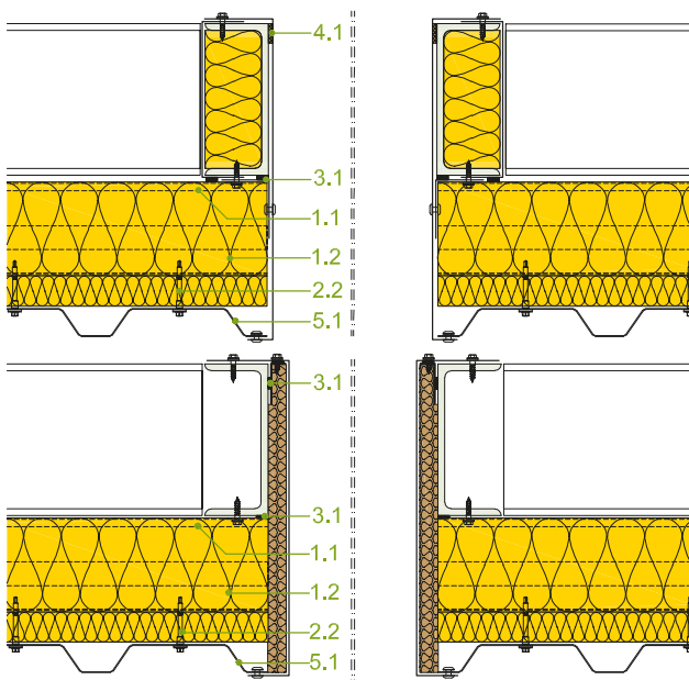
Seitliche Toranschlüsse
