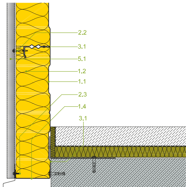
Sockelausbildung mit vorstehender Stahlkassette und Fußbodendämmung
